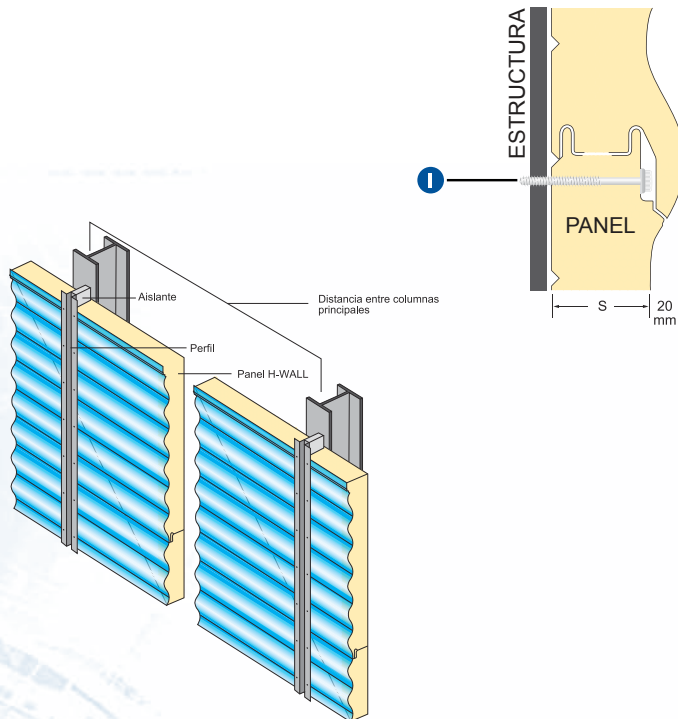
Detalle de la junta Longitudinal
