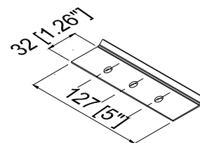
Clip de fijación muro
